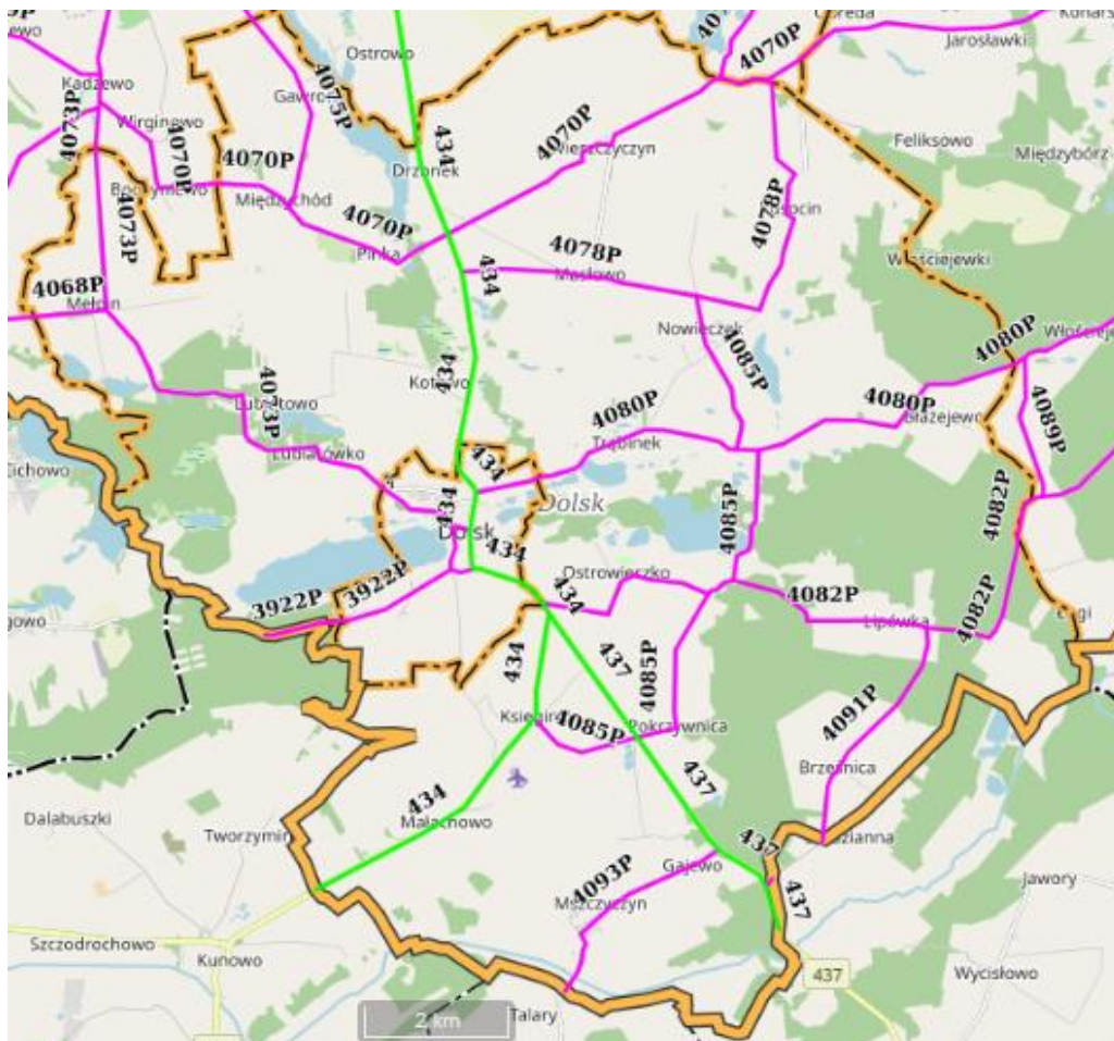
Rysunek 8 Sieć dróg powiatowych na terenie gminy Dolsk
