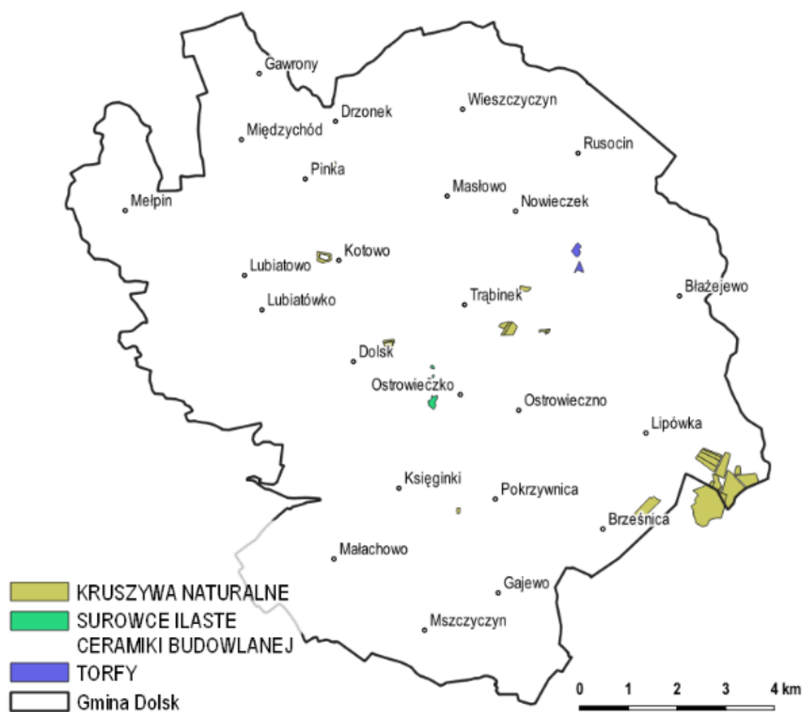
Rysunek 6 ZłoŜa surowców naturalnych na terenie gminy Dolsk
